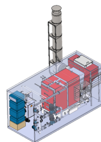
Компновка модуля
