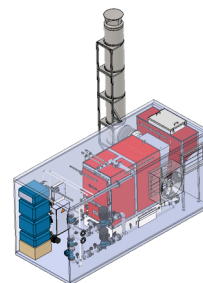
Компьютерная модель модуля
