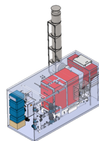
Компновка модуля
