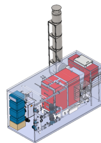
Компоновка модуля
